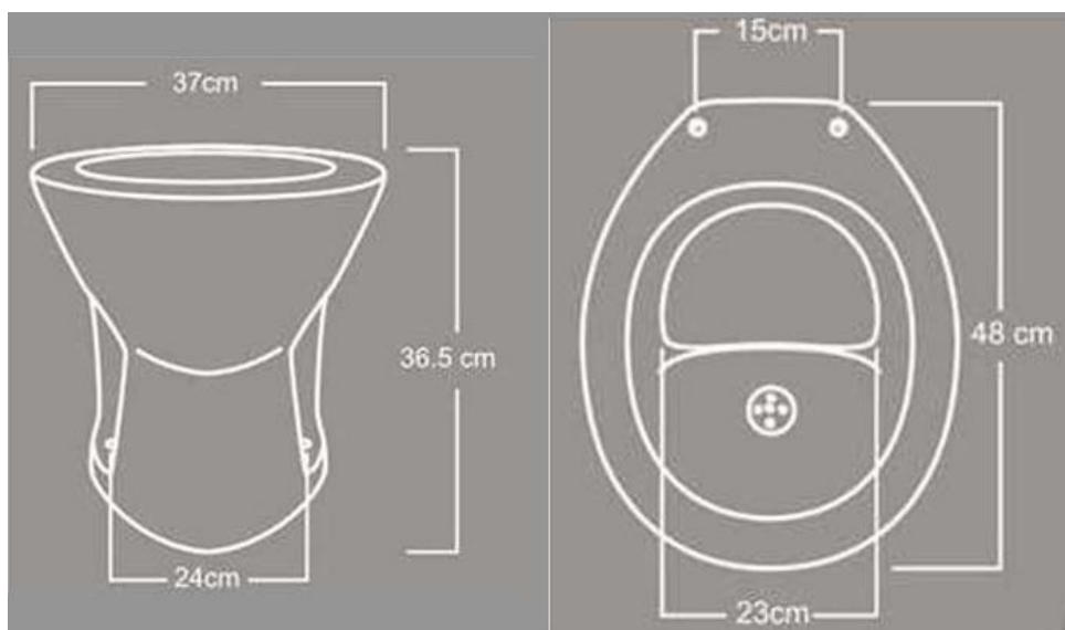
(Gráfico con las medidas del Inodoro)
